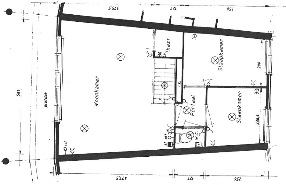
2 e verdieping
